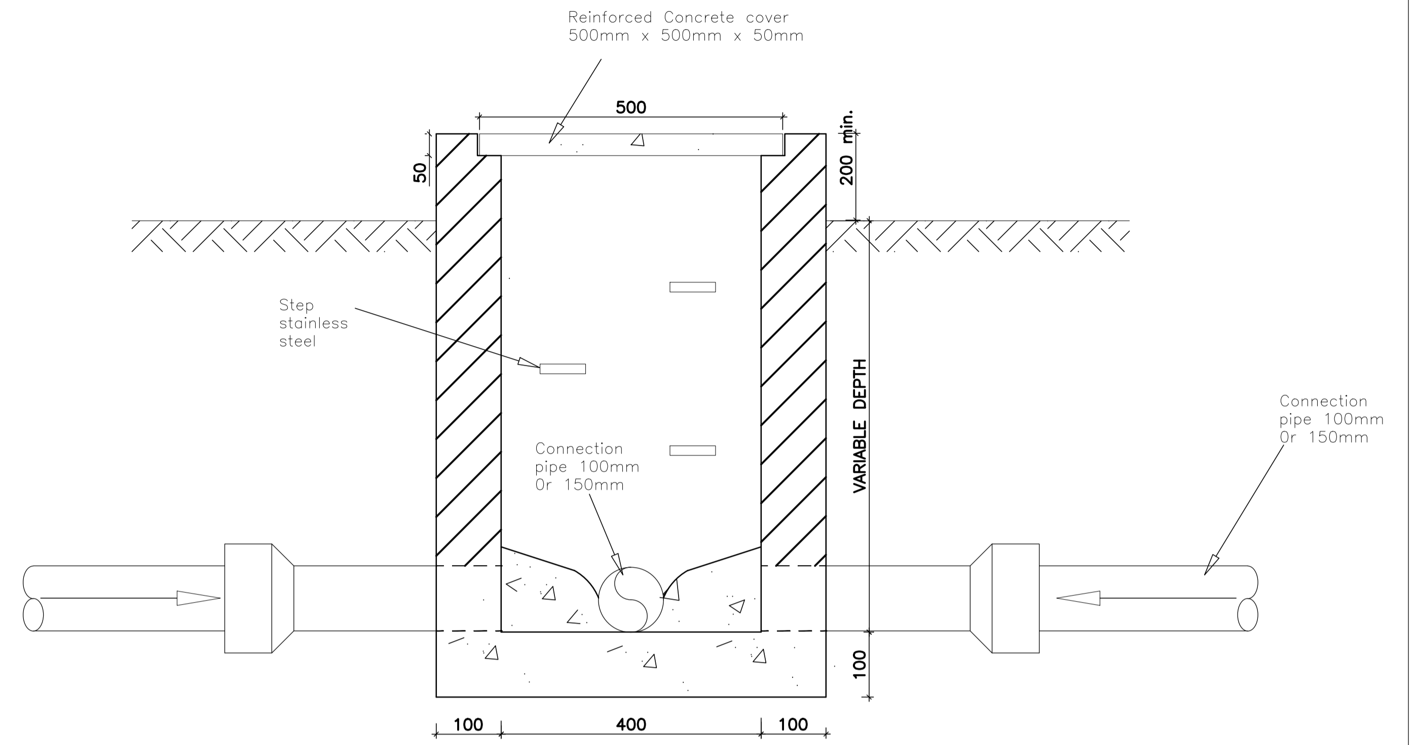
SECTION A-A
